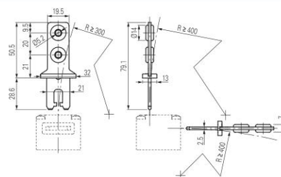
Actuador VF KEYF22
