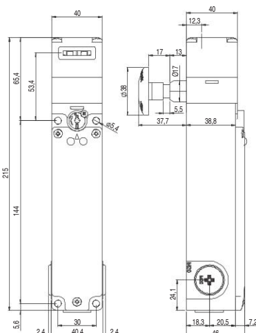
Interruptor FG 6•D7D•• Principio de funcionamiento D con desenclavamiento auxiliar sellable con plomo y pulsador de desbloqueo de emergencia
