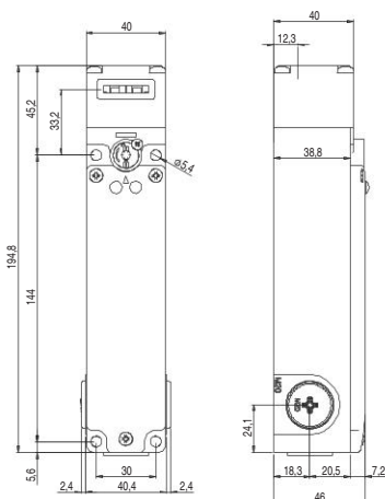
Interruptor FG 6•D6D•• Principio de funcionamiento D con desenclavamiento auxiliar por llave y pulsador de desbloqueo de emergencia
