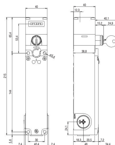
Interruptor FG 6•D7E•• Principio de funcionamiento E con pulsador de desbloqueo de emergencia
