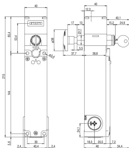
Interruptor FG 6•D6D•• Principio de funcionamiento D con desenclavamiento auxiliar por llave y pulsador de desbloqueo de emergencia
